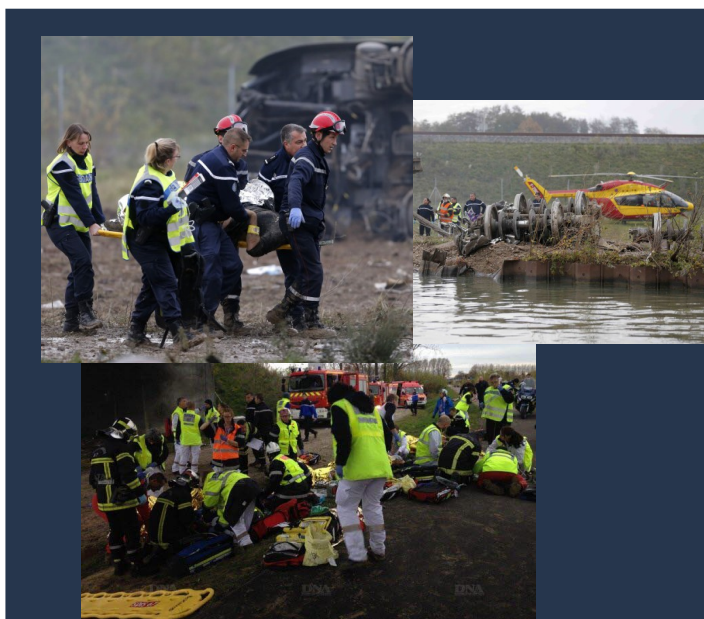
Accident de la rame d'essai du TGV Est le 14 novembre 2015 à Eckwersheim
